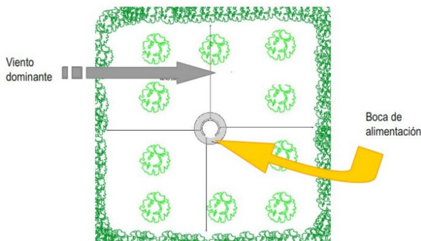
Posició de la boca d'alimentació d'un cremador agrícola respecte al vent dominant. Font: Norma Tècnica de Cremadors Agrícoles (PPIFD Polinyà del Xúquer).
