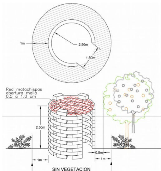
Planta i alçat d'un cremador degudament condicionat. Font: Norma Tècnica de Cremadors Agrícoles (PPIFD Polinyà del Xúquer).
