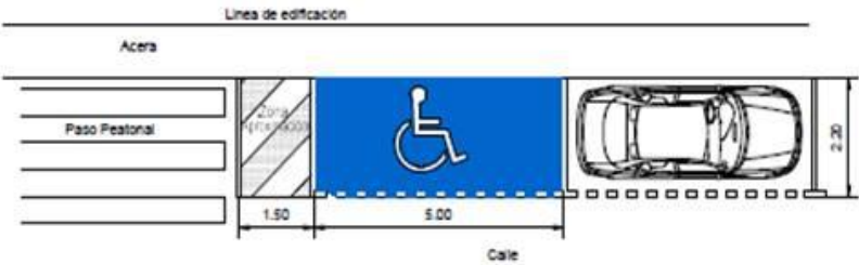
Figura 7. Plaza reservada en línea a la acera junto cruce peatonal
