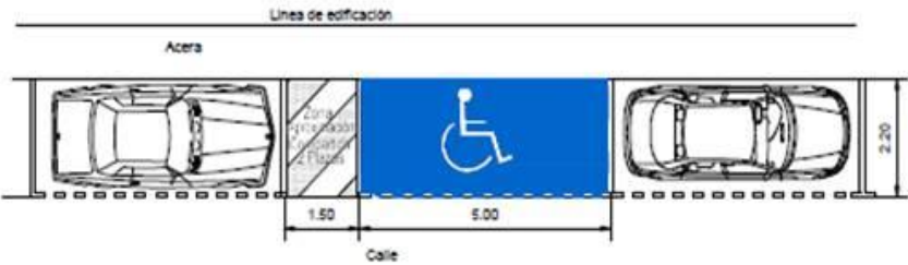
Figura 8. Plaza reservada en línea a la acera en espacio transferencia único
