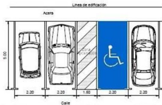
Figura 3. Plaza reservadas en perpendicular a la acera con espacio transferencia único
