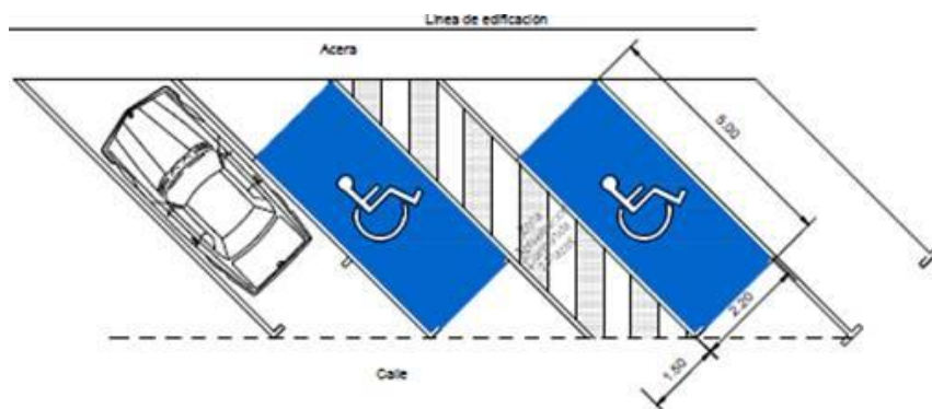
Figura 4 Plaza reservada en diagonal a la acera espacio transferencia compartido
