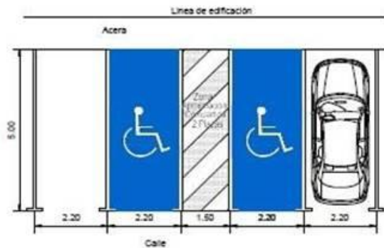
Figura 1. Plazas reservadas en perpendicular a la acera con espacio transferencia compartido
