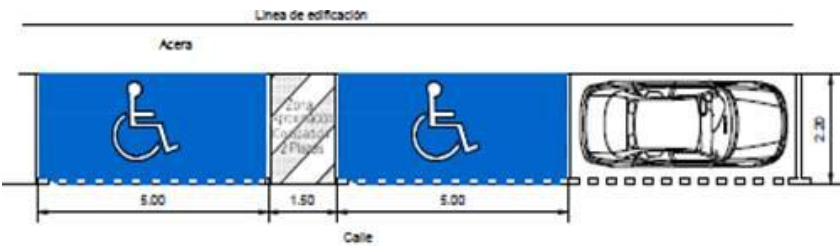
Figura 6. Plaza reservada en línea a la acera en espacio transferencia compartido
