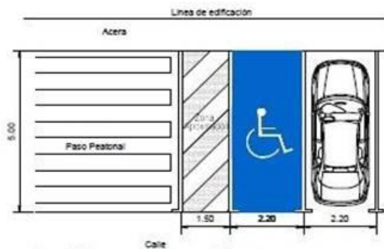
Figura 2. Plaza reservada en perpendicular a la acera junto cruce peatonal
