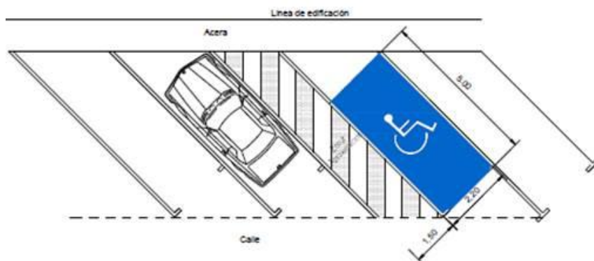
figura 5. Plaza reservada en diagonal a la acera espacio transferencia único
