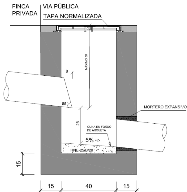
Arqueta tomamuestras 40 x 40. Cotas en cm.
