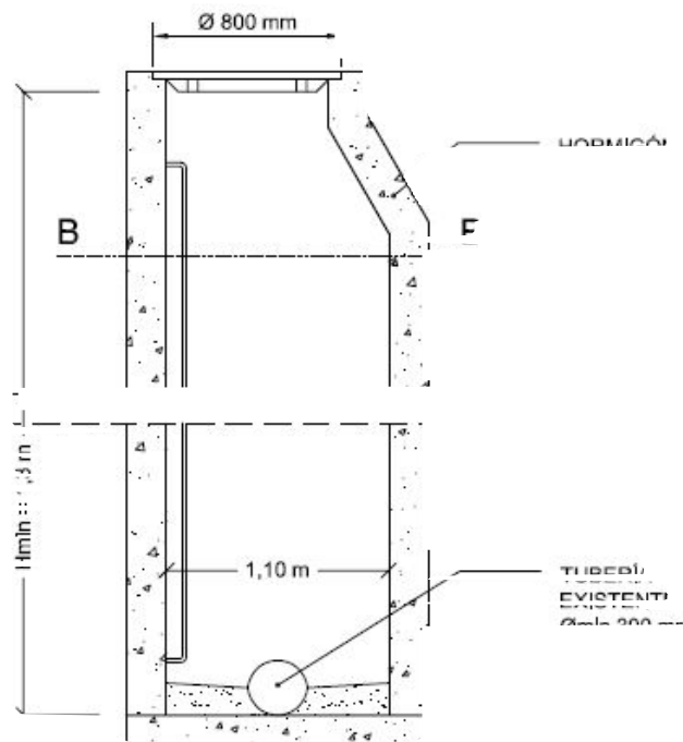
SECCIÓN A-A
