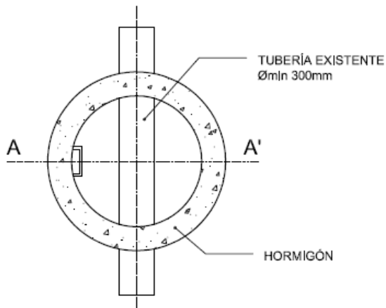
SECCIÓN B-B'
