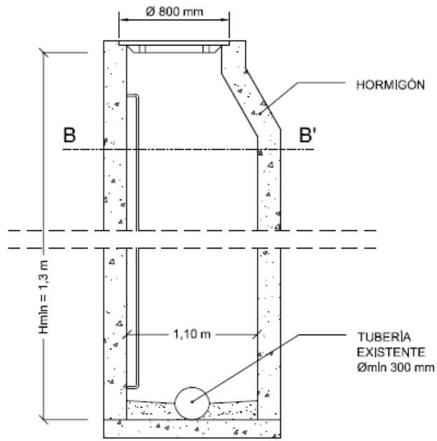
SECCIÓN A-A'
